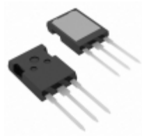
IXFX360N10T IXYS MOSFET N-CH 100V 360A PLUS247
