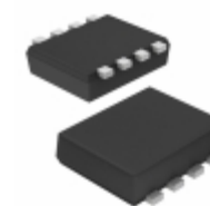
QS8K2TR Rohm Semiconductor MOSFET 2N-CH 30V 3.5A TSMT8
