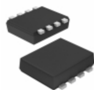
QS8K51TR Rohm Semiconductor MOSFET 2N-CH 30V 2A TSMT8
