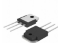
DPG60C400QB IXYS DIODE ARRAY GP 400V 30A TO3P
