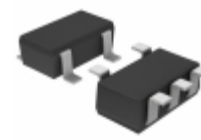
BU4822G-TR LAPIS Semiconductor IC VOLT DETECTOR 2.2V SSOP5
