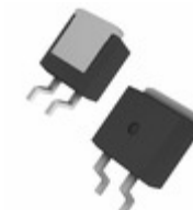
DSEP29-06AS-TUBE IXYS DIODE GEN PURP 600V 30A TO263
